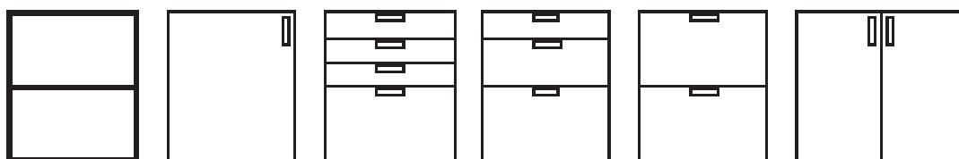
Underskabe Højde: 704 mm Bredde: 300, 400, 500 600, 800 cm (2 låger)
